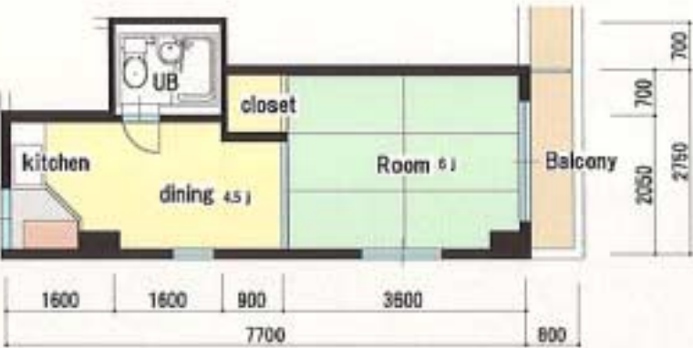
間取り
