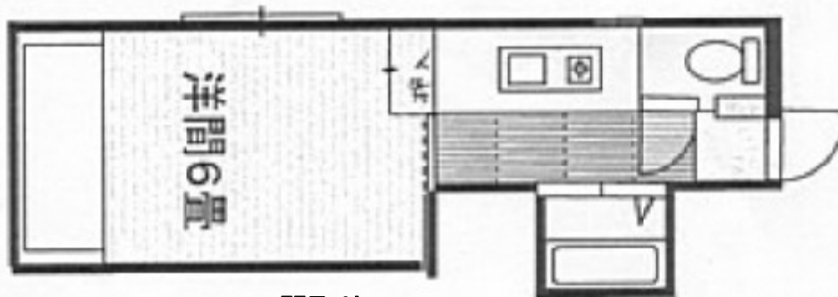
間取り
